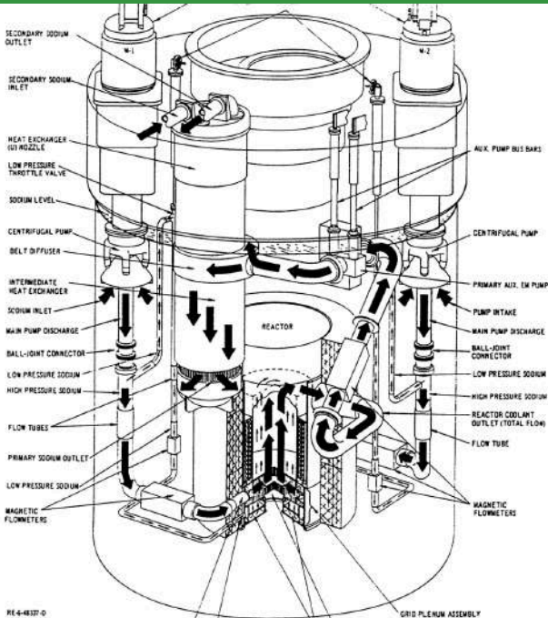
EBR-II reaktör kabının çizimi
